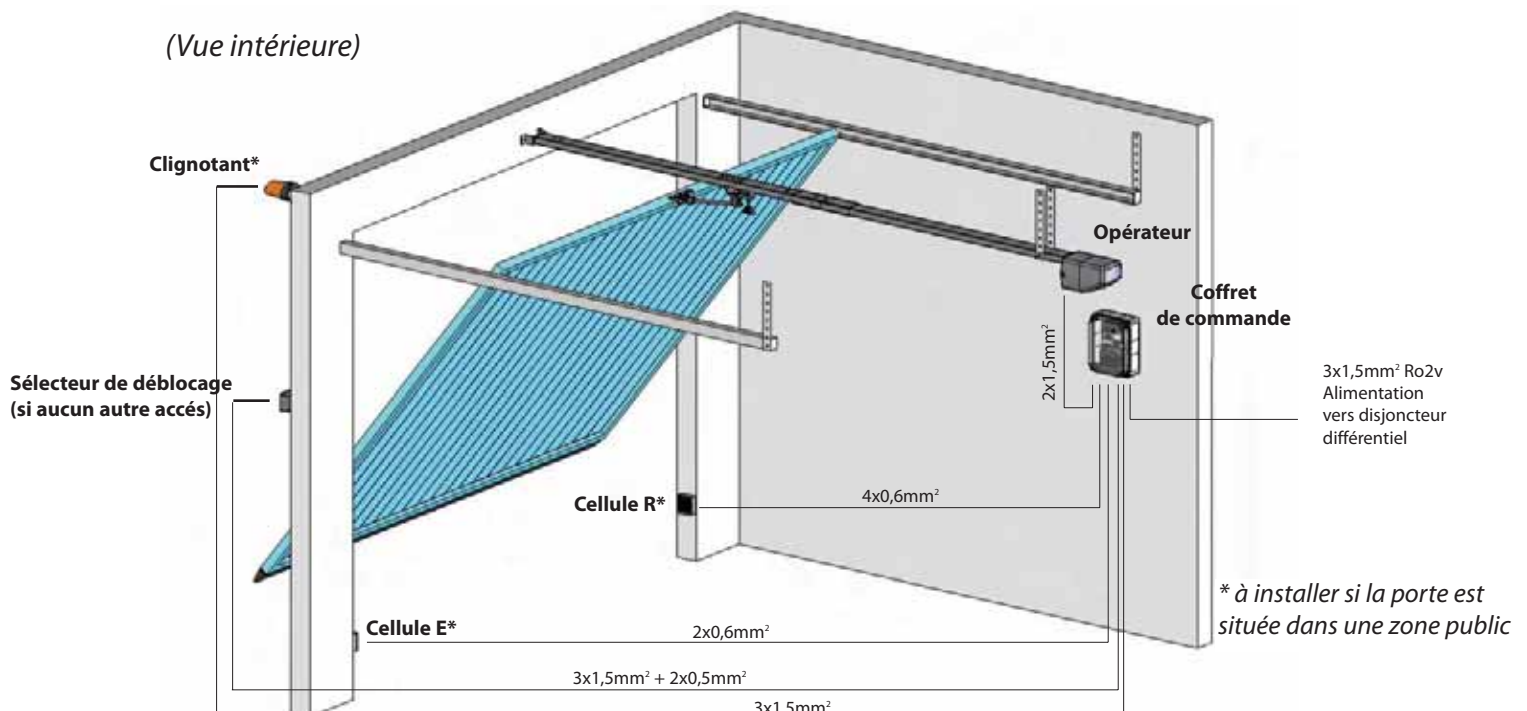
porte basculante débordante
